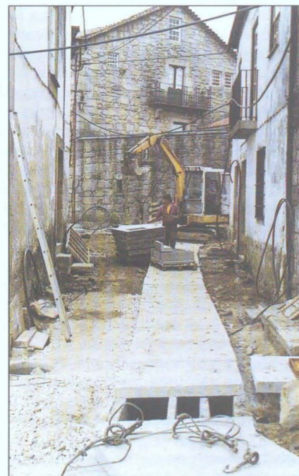
Pormenor do fecho da vala técnica na Travessa das Neves
