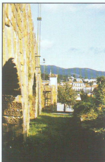
Ponte romana - colocação de escada metálica de acesso ao passeio marginal da margem direita do rio
